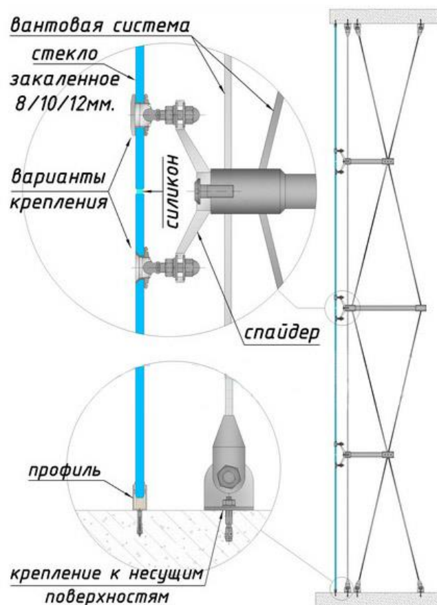
Рисунок 5.10 – Фрагмент вантового остекления
