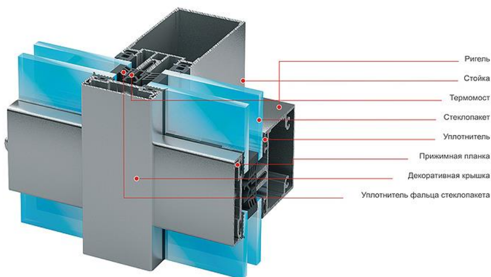
Рисунок 5.4 – Стоечно-ригельная система
