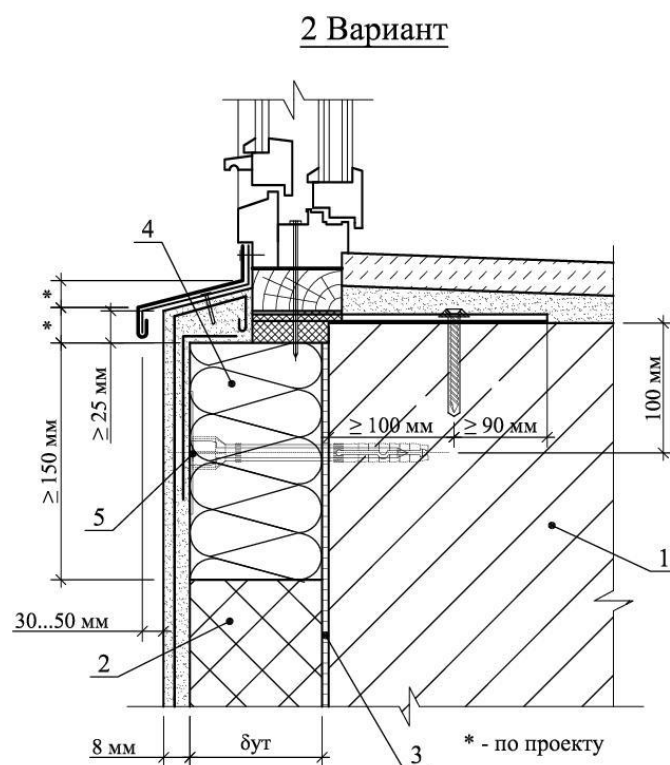
Рисунок 5.21 Пример примыкания конструкций фасадной системы без вентилируемого пространства к верхнему откосу оконного проема.
