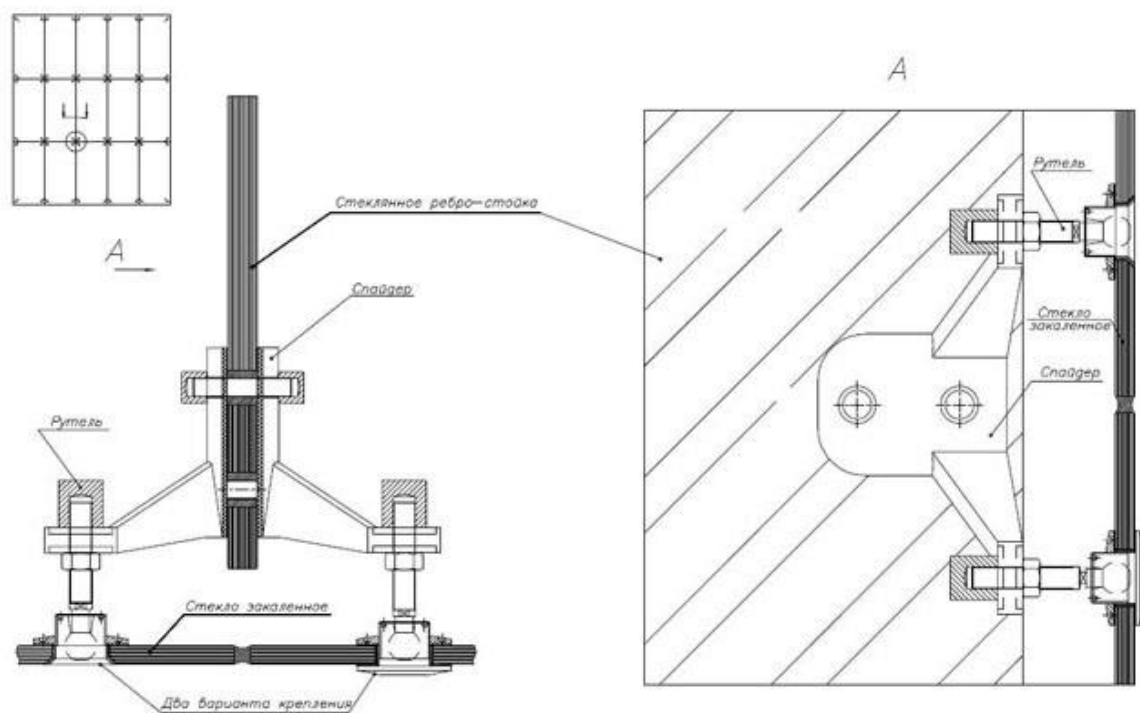
Рисунок 5.8 – Фрагмент спайдерного крепления фасада
