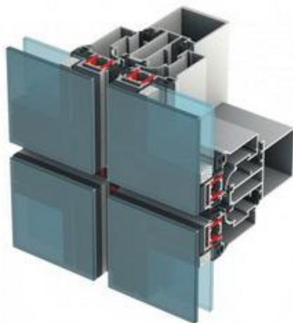
Рисунок 5.6 – Фрагмент структурного остекления
